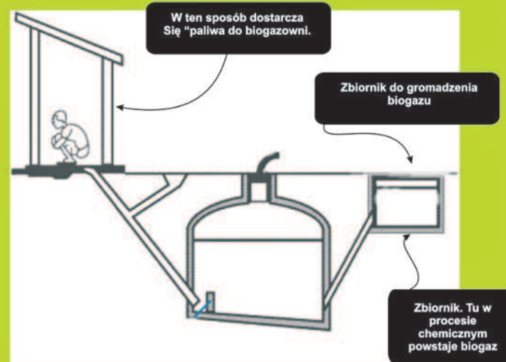
Schemat prostej biogazowni chińskiej
